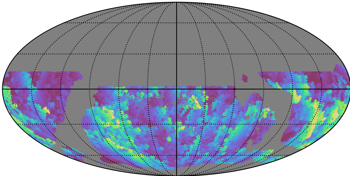
mw_roll_bulge_v3.3_10yrs WFD u band: Max normairmass
