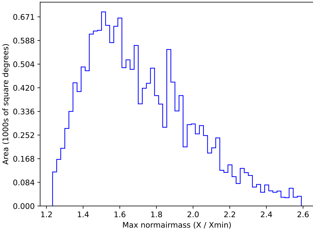
mw_roll_bulge_v3.3_10yrs WFD u band: Max normairmass
