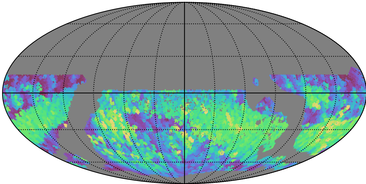
mw_roll_bulge_v3.3_10yrs WFD r band: Max normairmass
