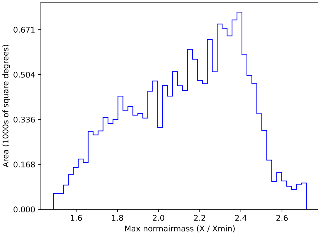
mw_roll_bulge_v3.3_10yrs WFD r band: Max normairmass
