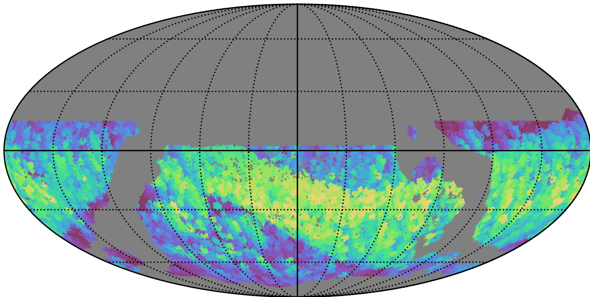
mw_roll_bulge_v3.3_10yrs WFD i band: Max normairmass
