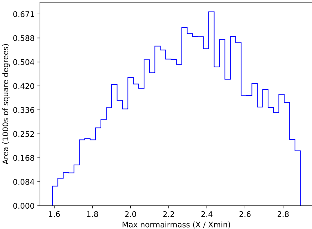
mw_roll_bulge_v3.3_10yrs WFD i band: Max normairmass
