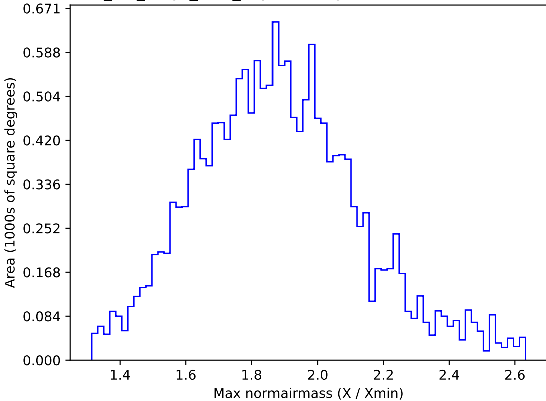
mw_roll_bulge_v3.3_10yrs WFD g band: Max normairmass
