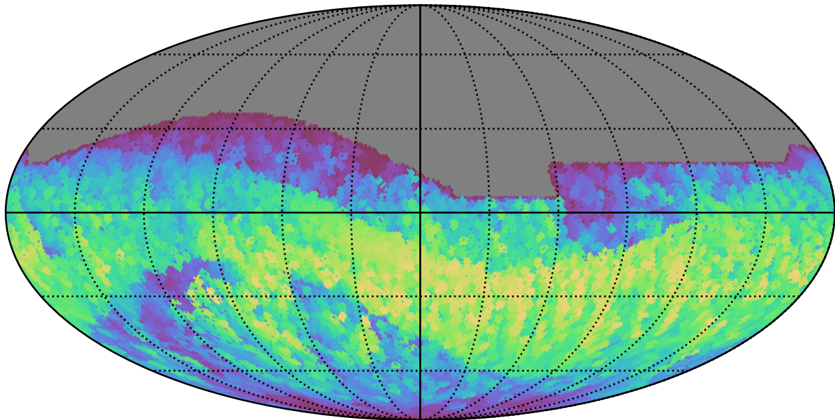
mw_roll_bulge_v3.3_10yrs All sky z band: Max normairmass
