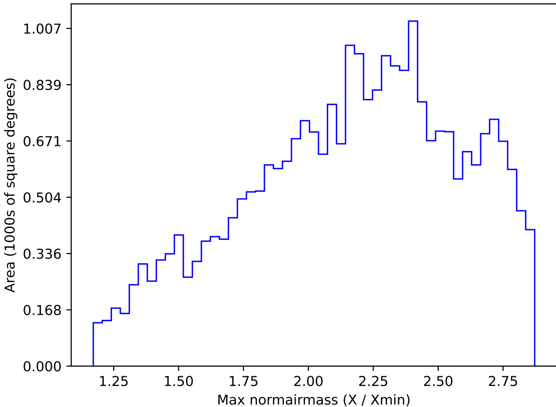
mw_roll_bulge_v3.3_10yrs All sky z band: Max normairmass
