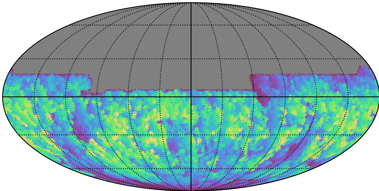
mw_roll_bulge_v3.3_10yrs All sky y band: Max normairmass
