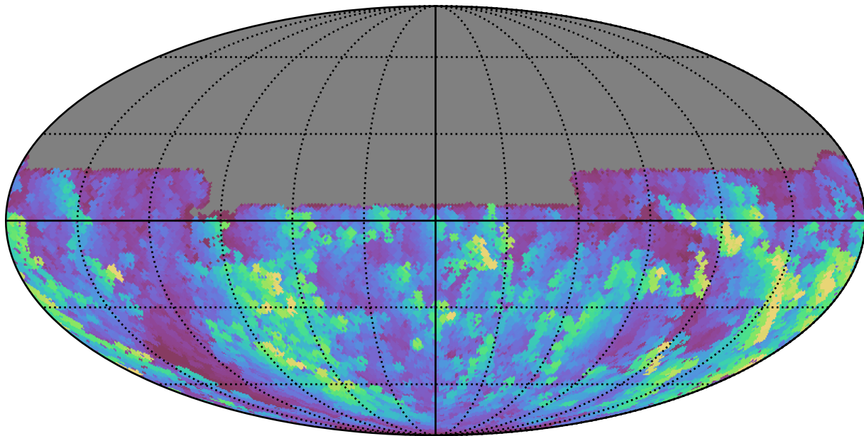
mw_roll_bulge_v3.3_10yrs All sky u band: Max normairmass
