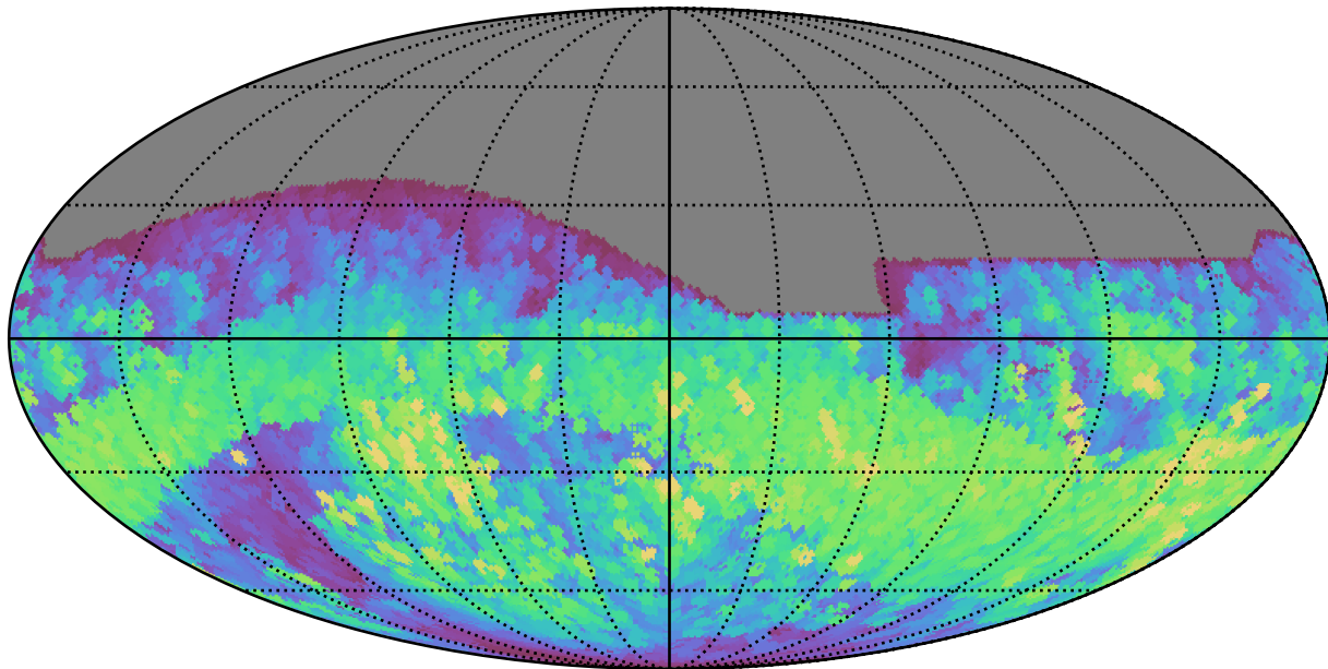
mw_roll_bulge_v3.3_10yrs All sky r band: Max normairmass
