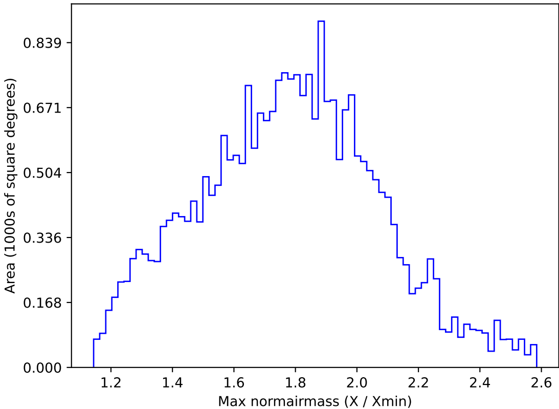
mw_roll_bulge_v3.3_10yrs All sky g band: Max normairmass
