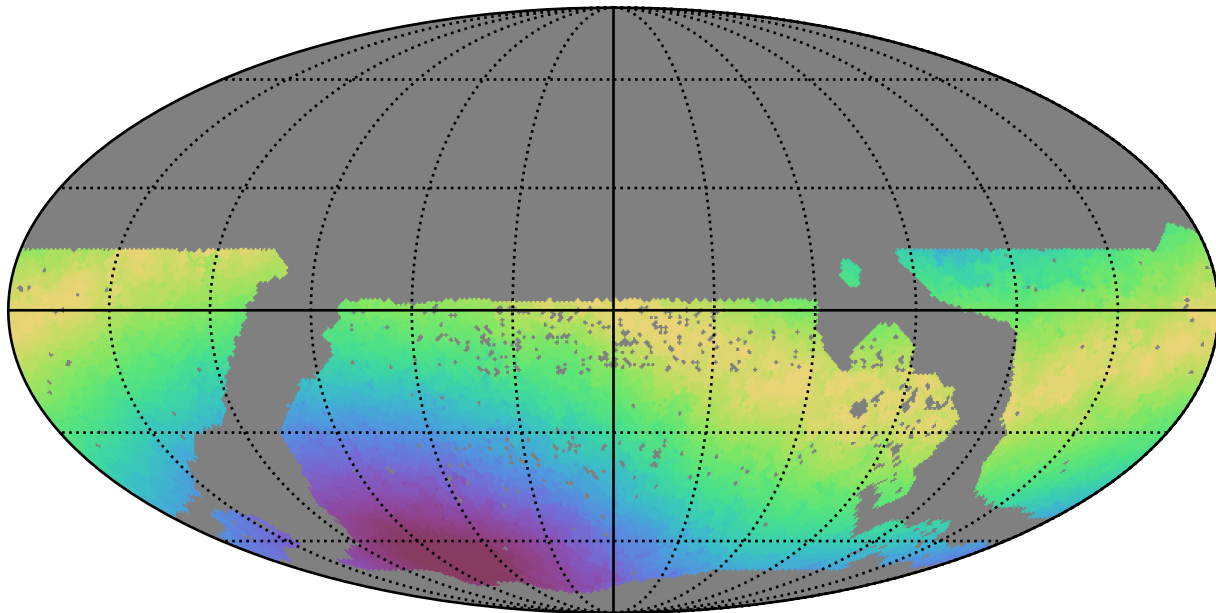
mw_roll_bulge_v3.3_10yrs WFD z band: Max moonDistance
