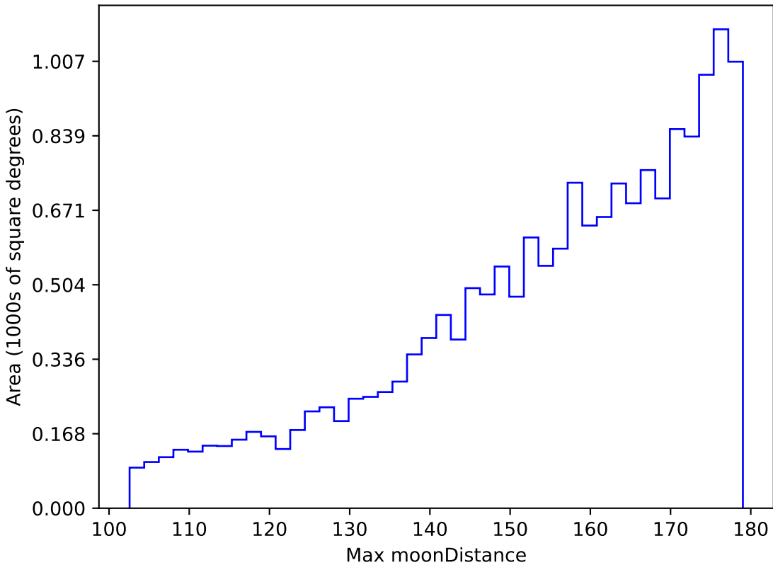
mw_roll_bulge_v3.3_10yrs WFD z band: Max moonDistance
