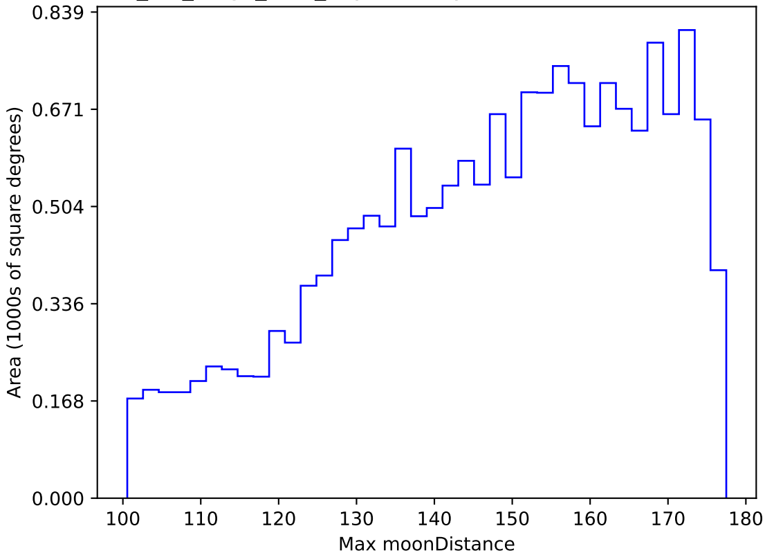
mw_roll_bulge_v3.3_10yrs WFD y band: Max moonDistance
