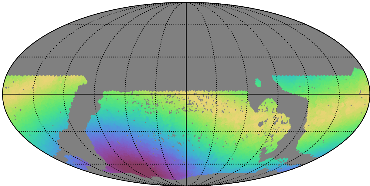
mw_roll_bulge_v3.3_10yrs WFD i band: Max moonDistance
