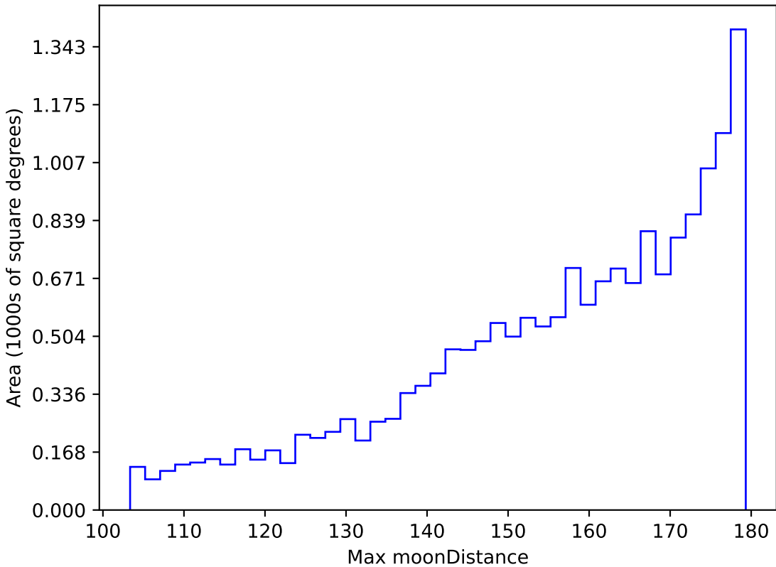
mw_roll_bulge_v3.3_10yrs WFD i band: Max moonDistance
