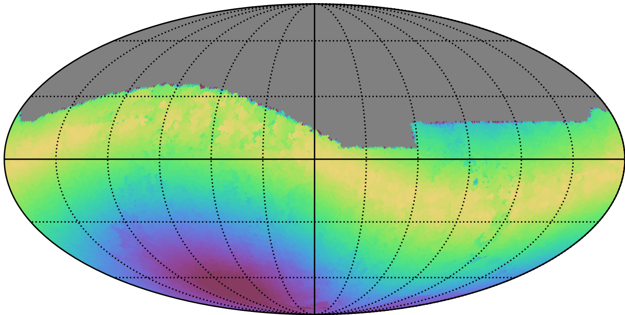
mw_roll_bulge_v3.3_10yrs All sky i band: Max moonDistance
