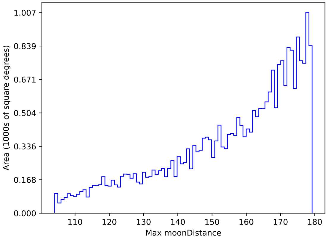
mw_roll_bulge_v3.3_10yrs All sky i band: Max moonDistance
