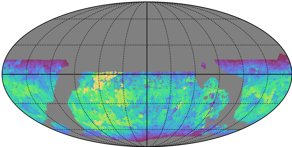
mw_roll_bulge_v3.3_10yrs WFD y band: Max fiveSigmaDepth
