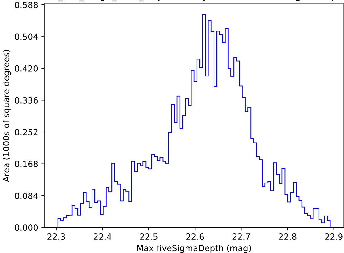
mw_roll_bulge_v3.3_10yrs WFD y band: Max fiveSigmaDepth
