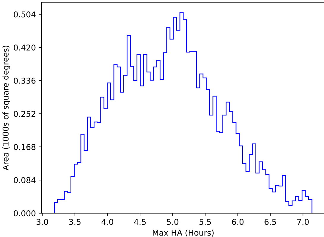
mw_roll_bulge_v3.3_10yrs WFD z band: Max HA
