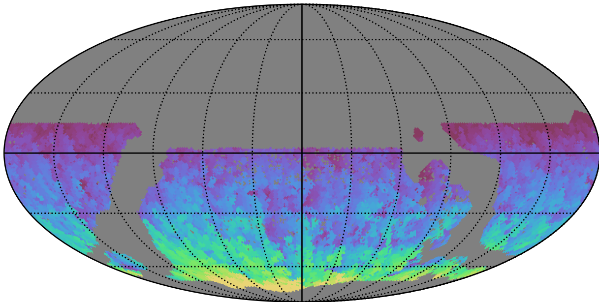
mw_roll_bulge_v3.3_10yrs WFD y band: Max HA
