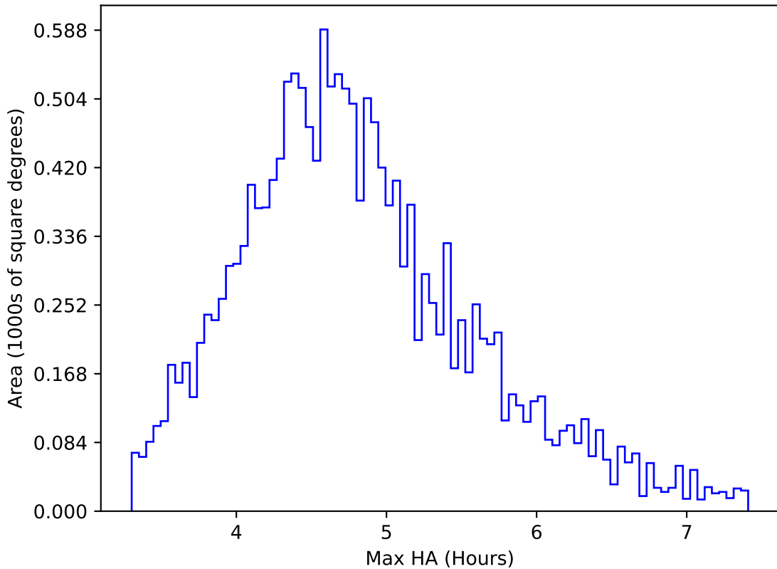
mw_roll_bulge_v3.3_10yrs WFD y band: Max HA
