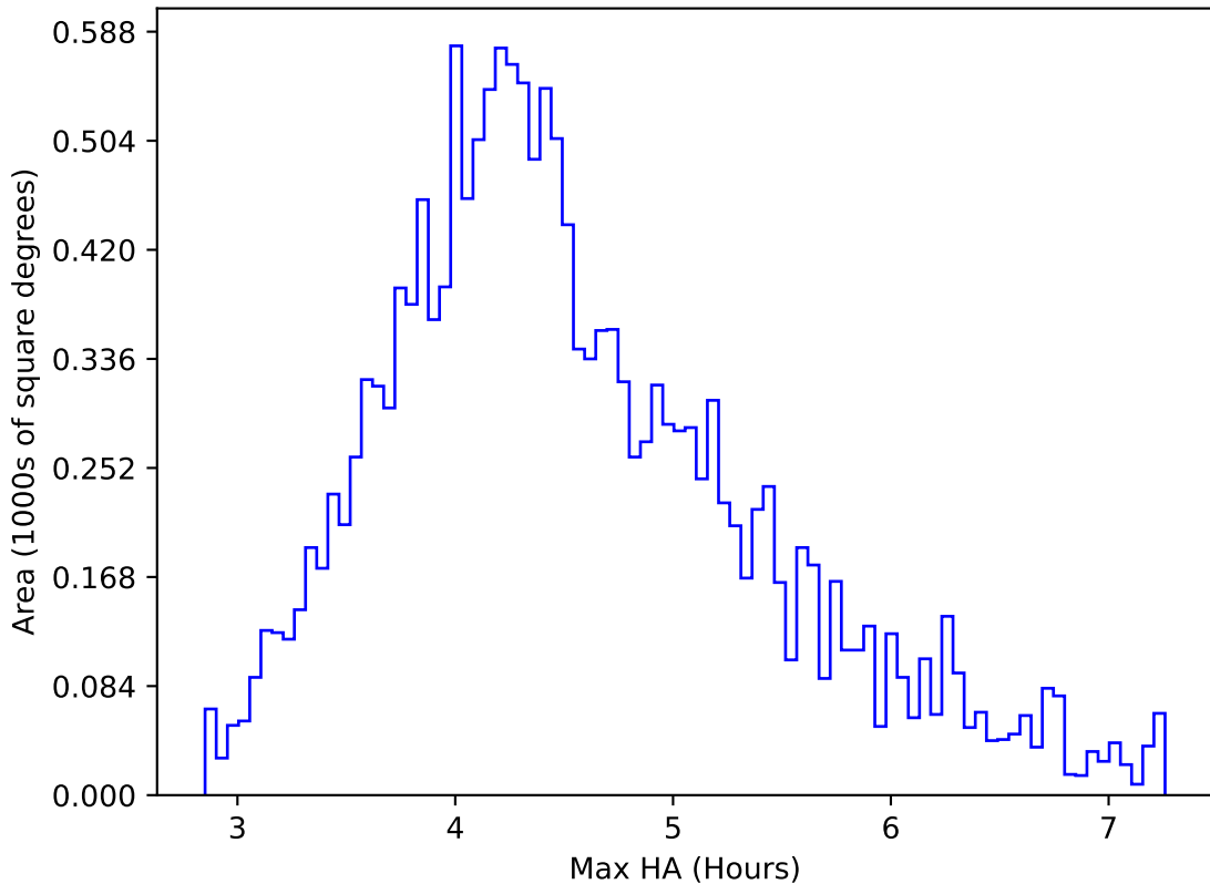
mw_roll_bulge_v3.3_10yrs WFD r band: Max HA
