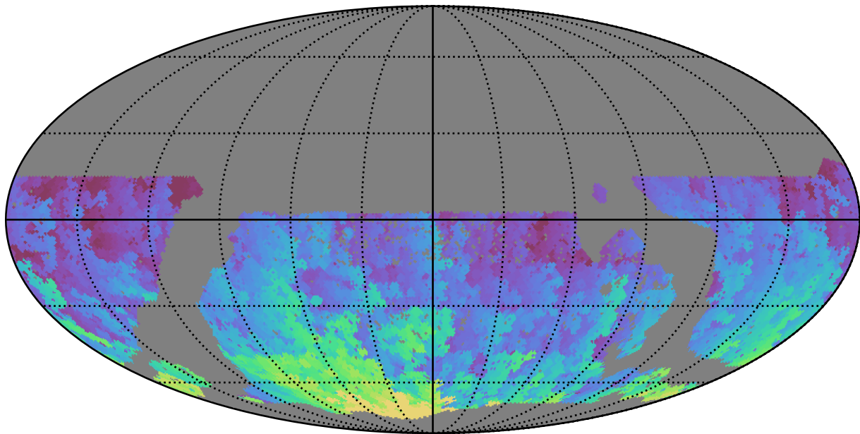
mw_roll_bulge_v3.3_10yrs WFD g band: Max HA
