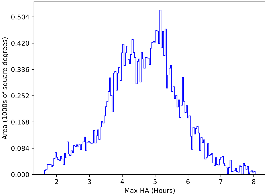
mw_roll_bulge_v3.3_10yrs All sky z band: Max HA
