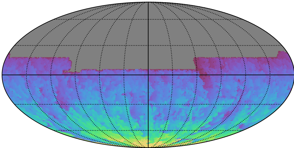
mw_roll_bulge_v3.3_10yrs All sky y band: Max HA
