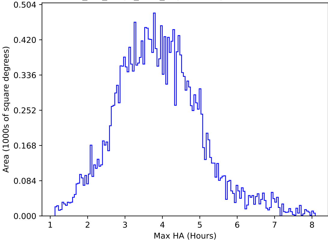
mw_roll_bulge_v3.3_10yrs All sky u band: Max HA
