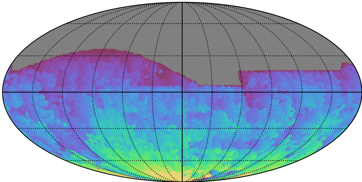
mw_roll_bulge_v3.3_10yrs All sky r band: Max HA
