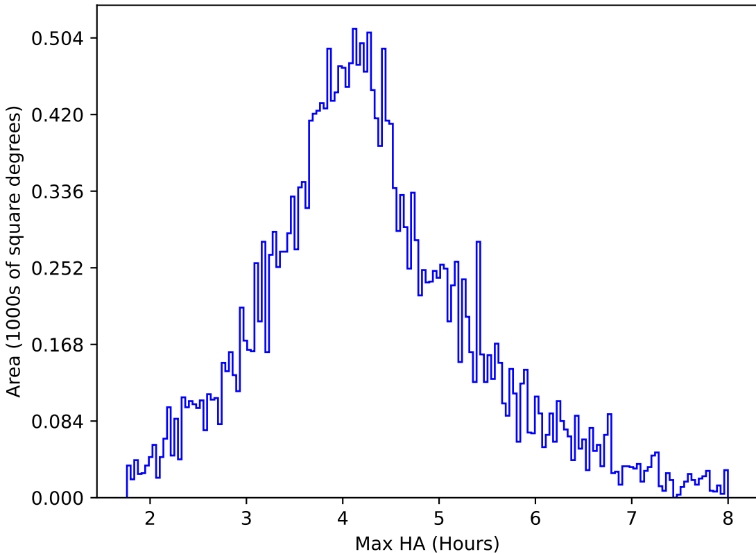
mw_roll_bulge_v3.3_10yrs All sky r band: Max HA
