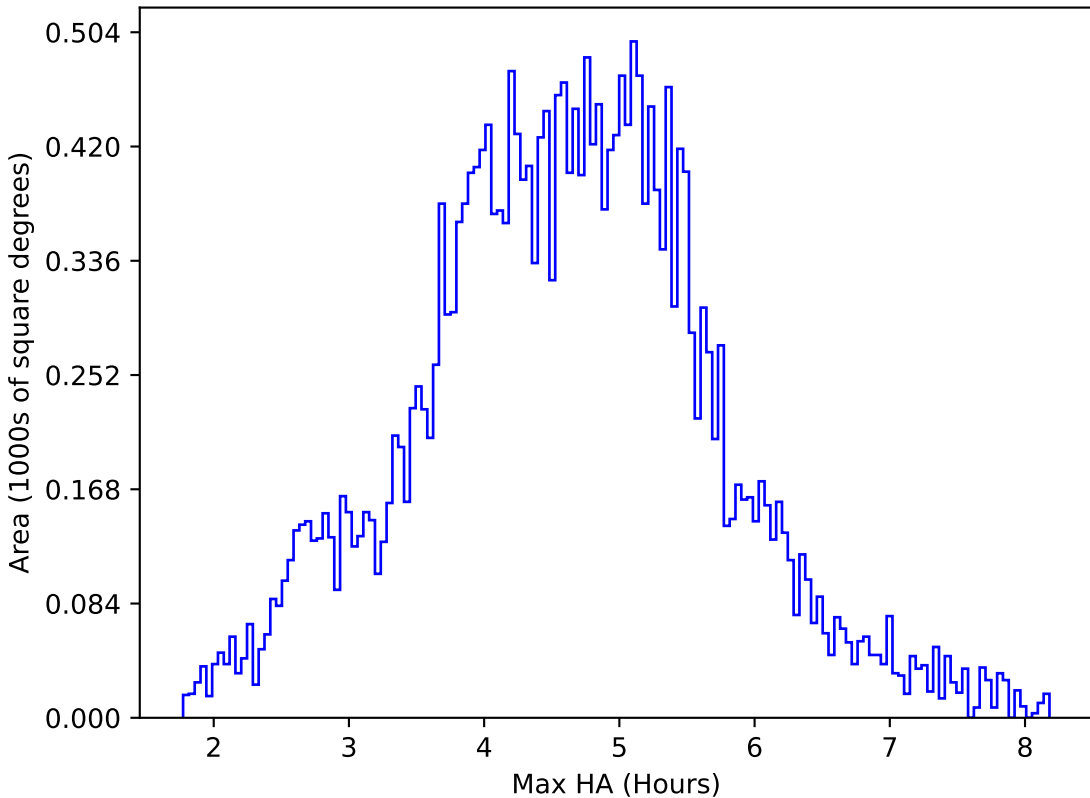
mw_roll_bulge_v3.3_10yrs All sky i band: Max HA
