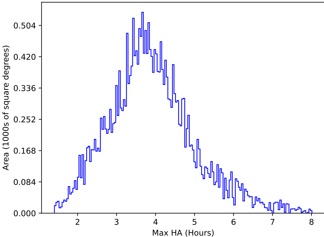
mw_roll_bulge_v3.3_10yrs All sky g band: Max HA
