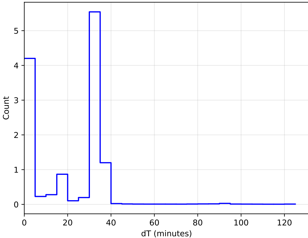
1e6 mw_roll_bulge_v3.3_10yrs All sky: DeltaT Histogram
