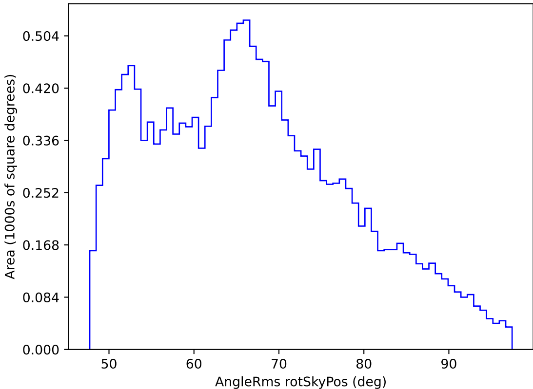
mw_roll_bulge_v3.3_10yrs WFD z band: AngleRms rotSkyPos
