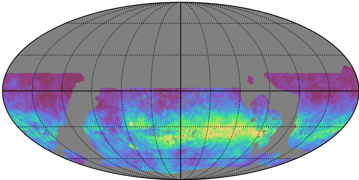
mw_roll_bulge_v3.3_10yrs WFD y band: AngleRms rotSkyPos
