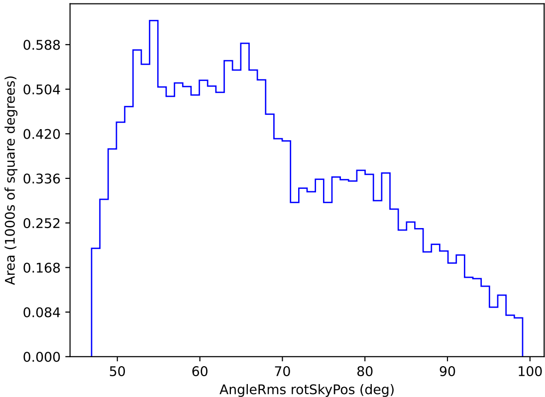
mw_roll_bulge_v3.3_10yrs WFD r band: AngleRms rotSkyPos
