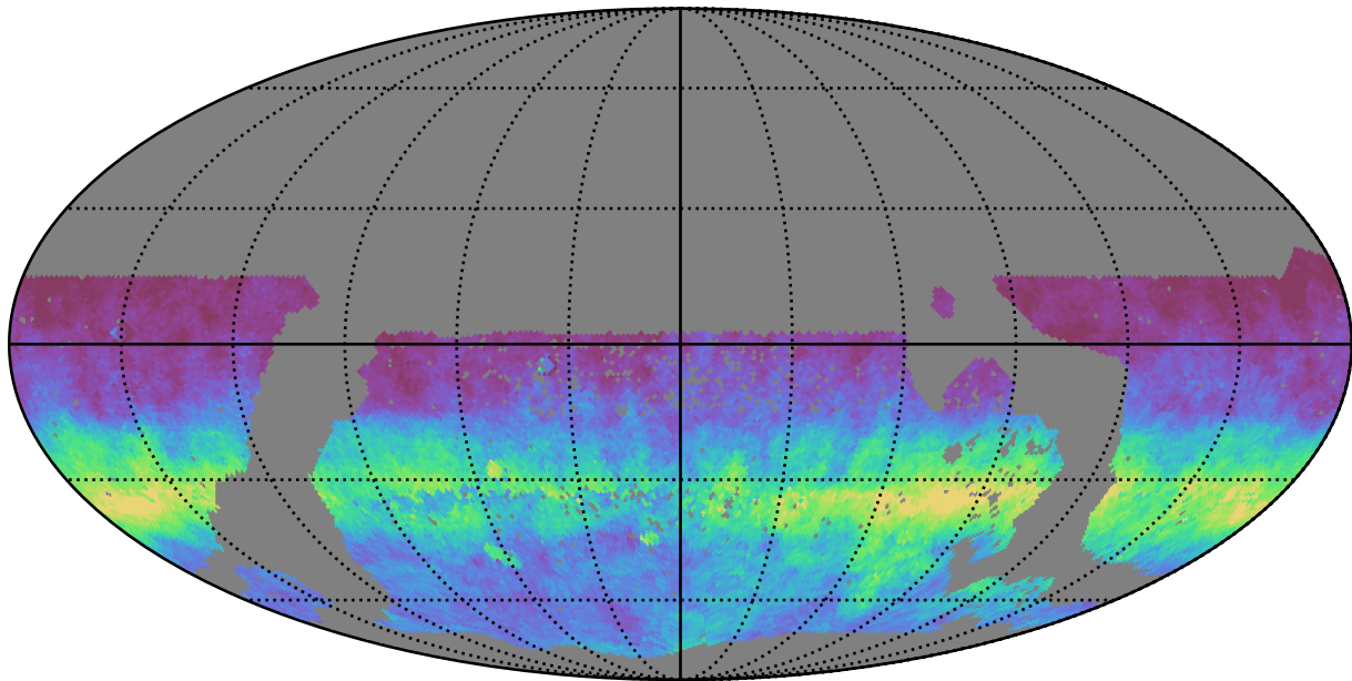
mw_roll_bulge_v3.3_10yrs WFD i band: AngleRms rotSkyPos
