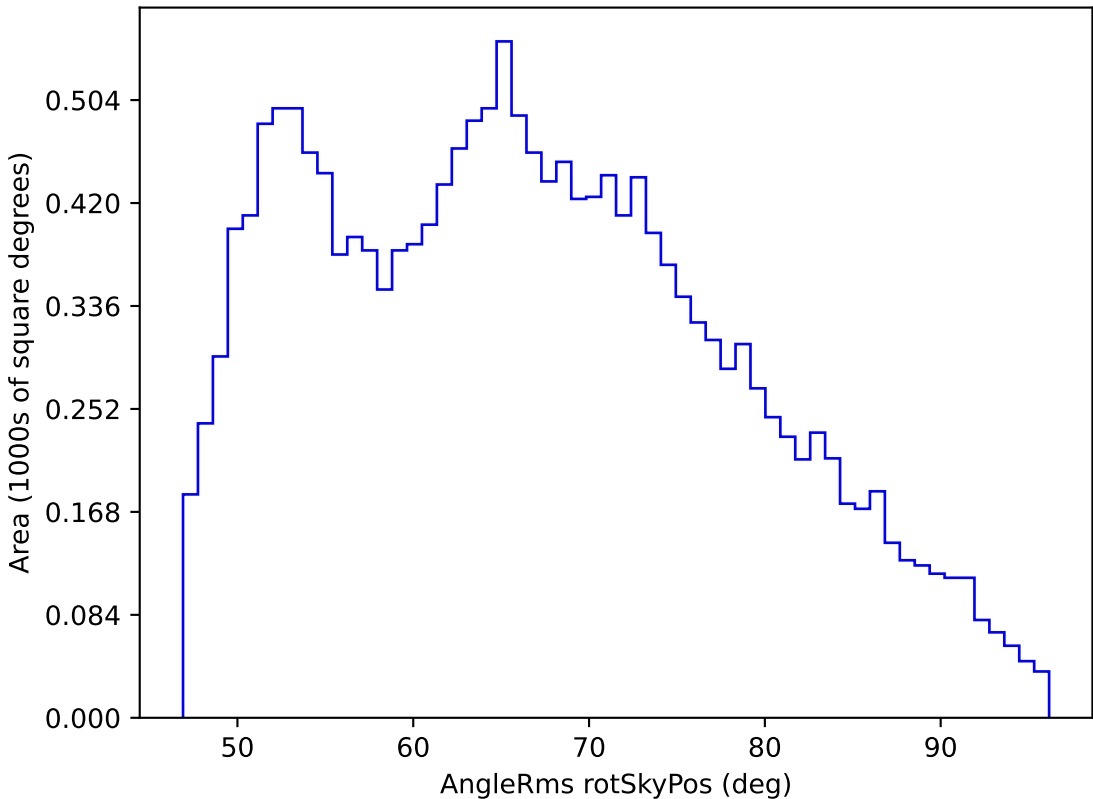
mw_roll_bulge_v3.3_10yrs WFD i band: AngleRms rotSkyPos
