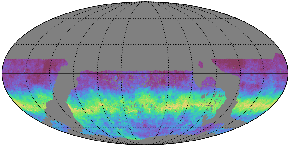
mw_roll_bulge_v3.3_10yrs WFD g band: AngleRms rotSkyPos
