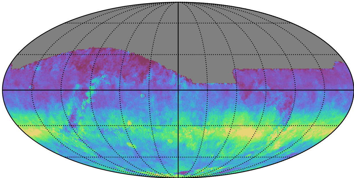
mw_roll_bulge_v3.3_10yrs All sky z band: AngleRms rotSkyPos
