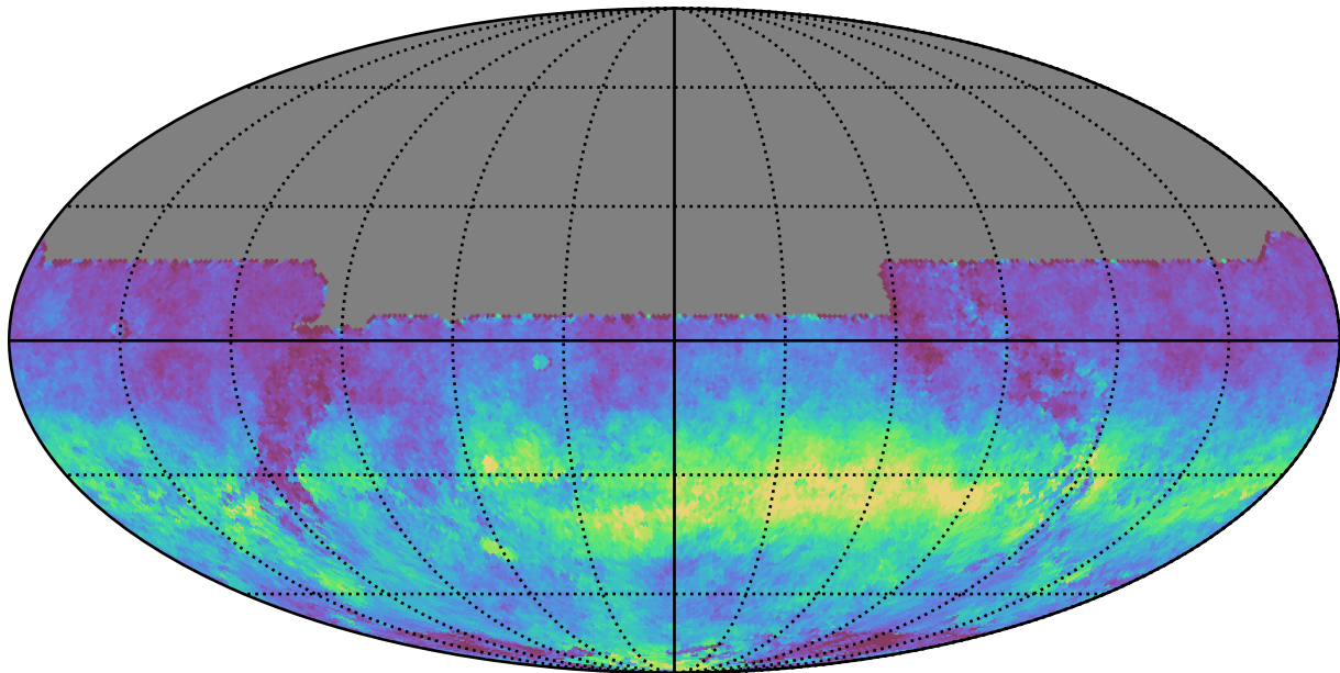
mw_roll_bulge_v3.3_10yrs All sky y band: AngleRms rotSkyPos
