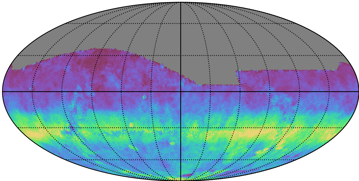
mw_roll_bulge_v3.3_10yrs All sky i band: AngleRms rotSkyPos
