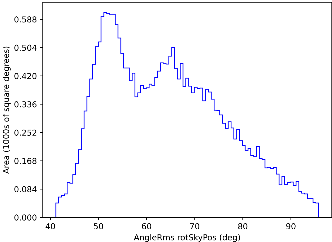
mw_roll_bulge_v3.3_10yrs All sky i band: AngleRms rotSkyPos
