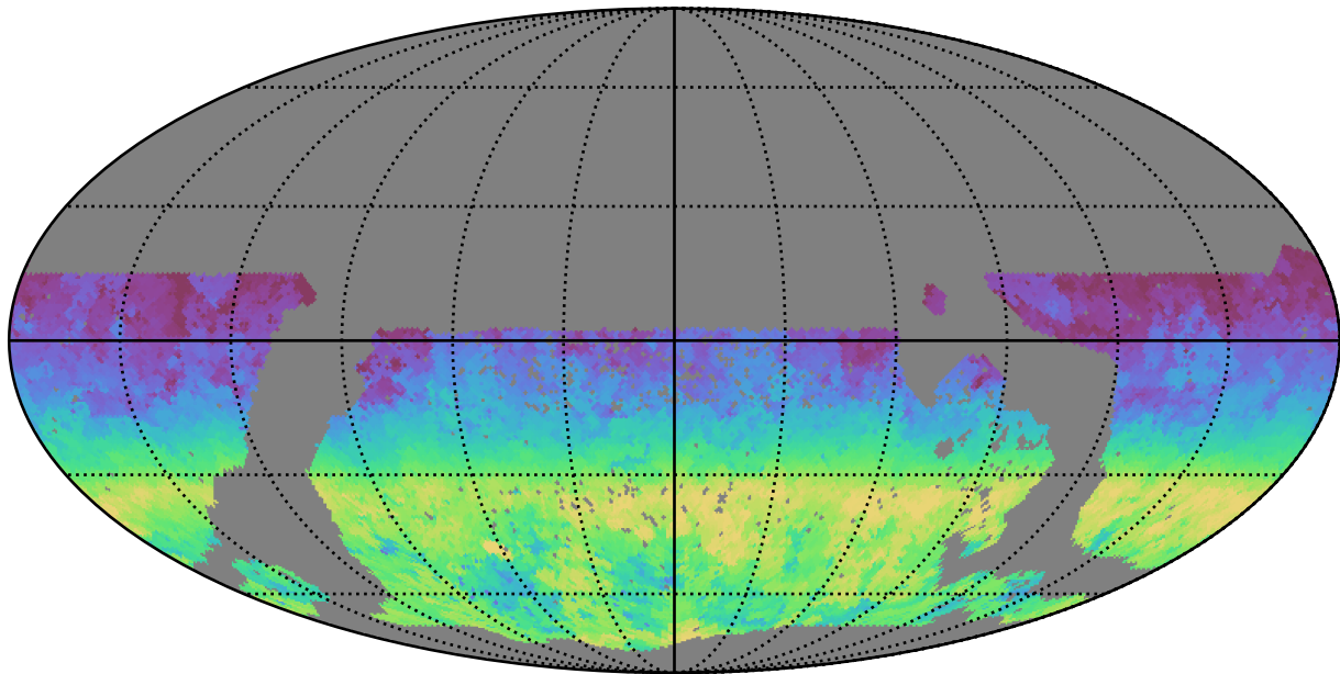
mw_roll_bulge_v3.3_10yrs WFD z band: AngleRange rotSkyPos
