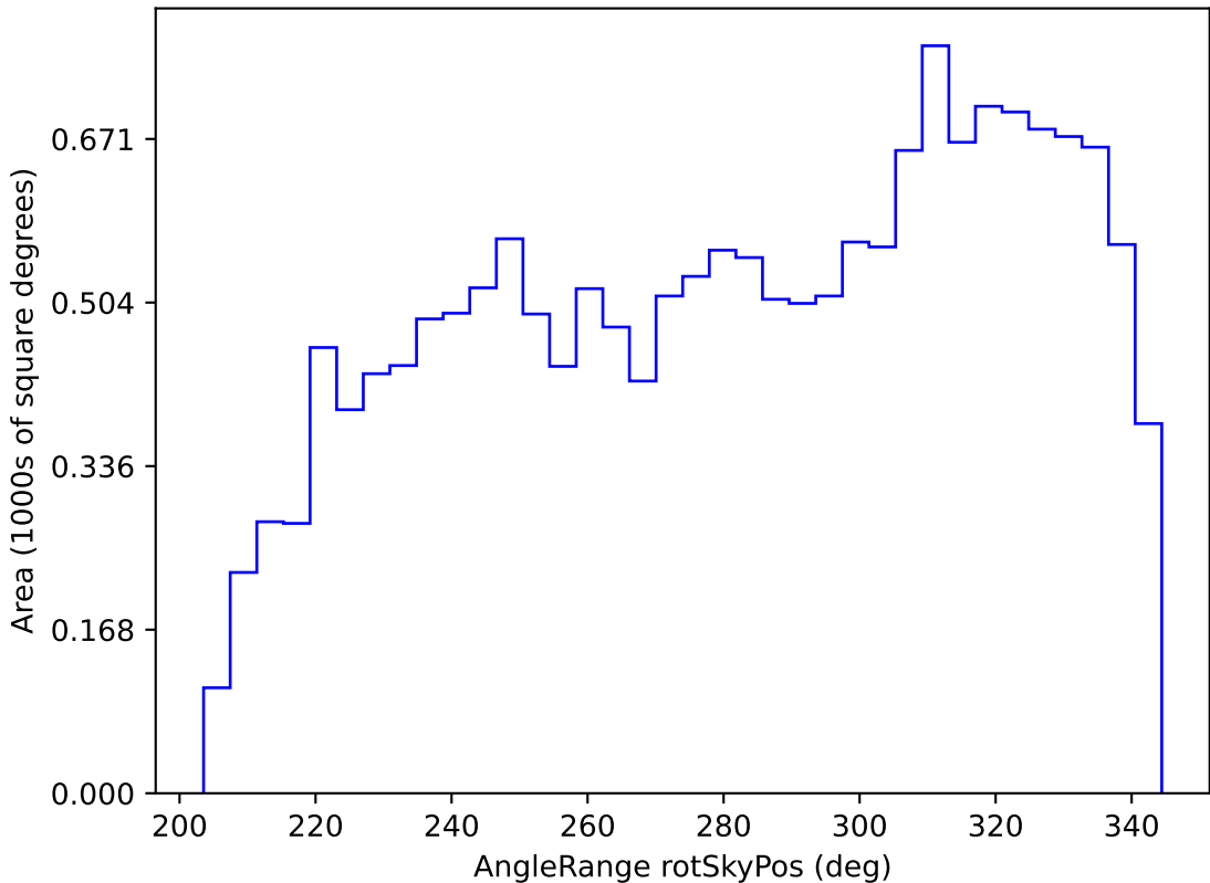
mw_roll_bulge_v3.3_10yrs WFD z band: AngleRange rotSkyPos
