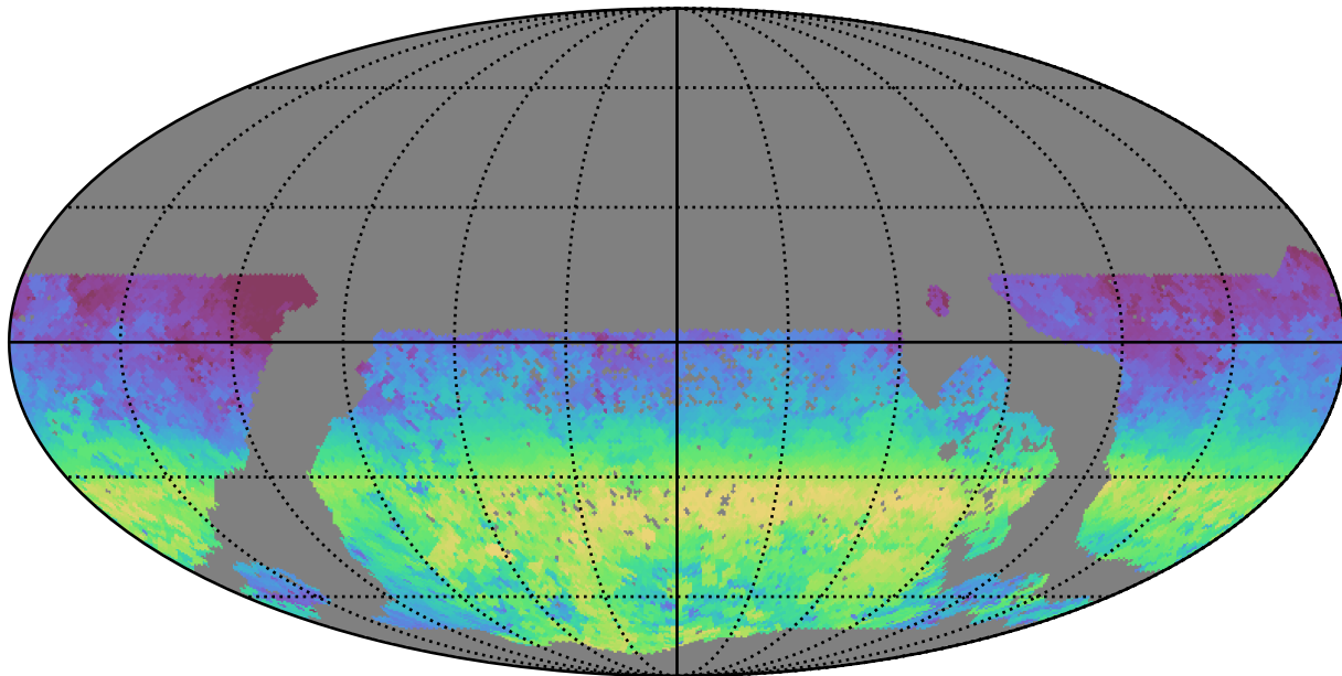
mw_roll_bulge_v3.3_10yrs WFD y band: AngleRange rotSkyPos
