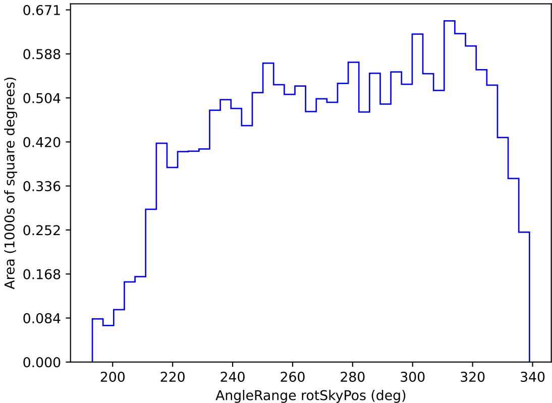
mw_roll_bulge_v3.3_10yrs WFD y band: AngleRange rotSkyPos
