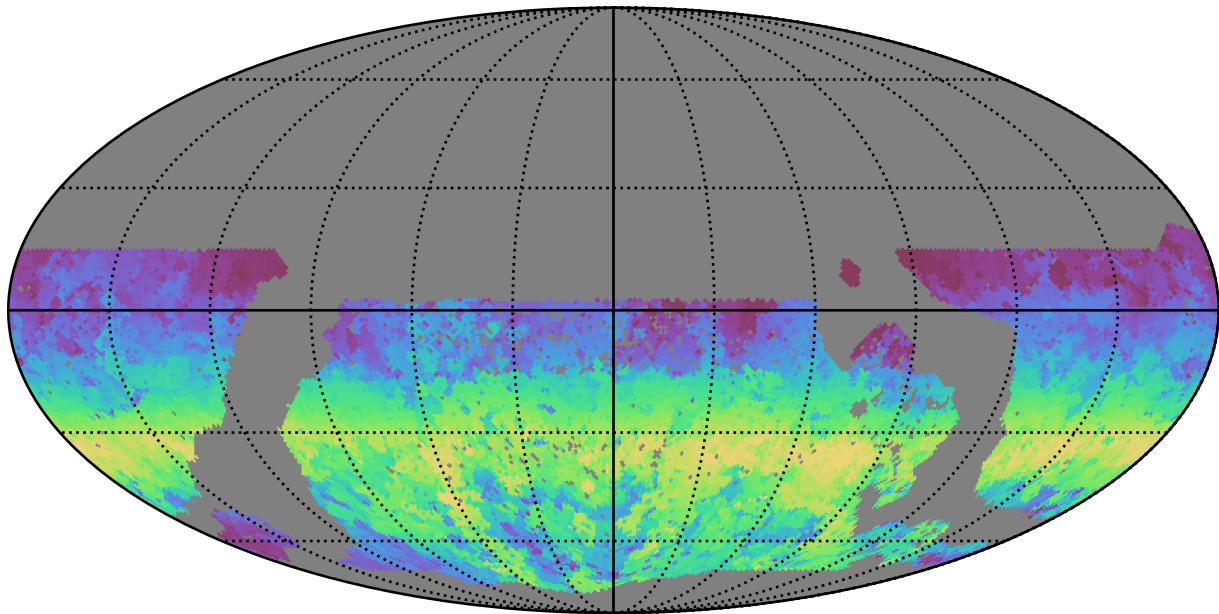
mw_roll_bulge_v3.3_10yrs WFD u band: AngleRange rotSkyPos
